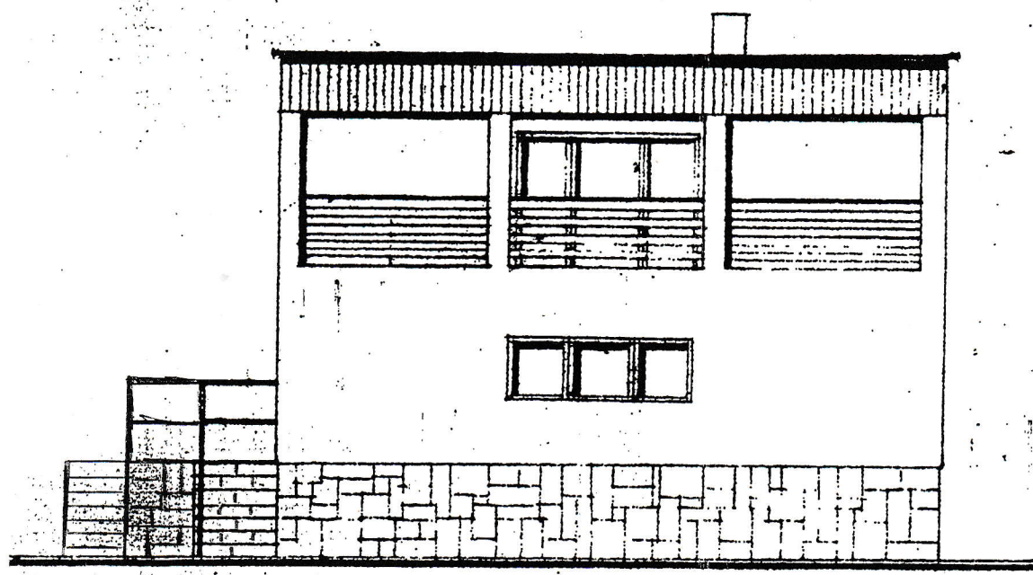
POHLED JIHOZÁPADNÍ
