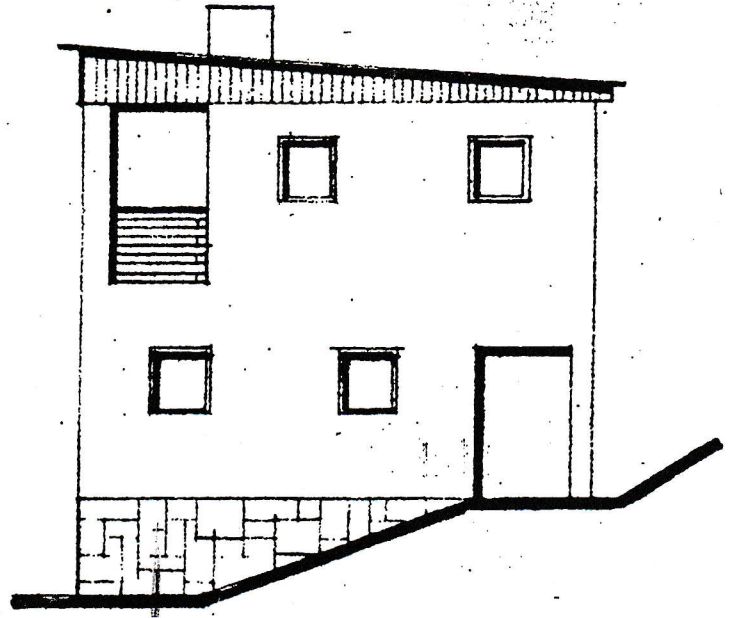
POHLED SV
